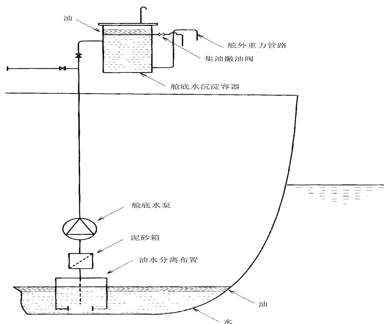
圖 2.2.5.3 (1) — 組合油水分離佈置與艙底水沉澱櫃 — 僅用於 400 總噸以下的小船
