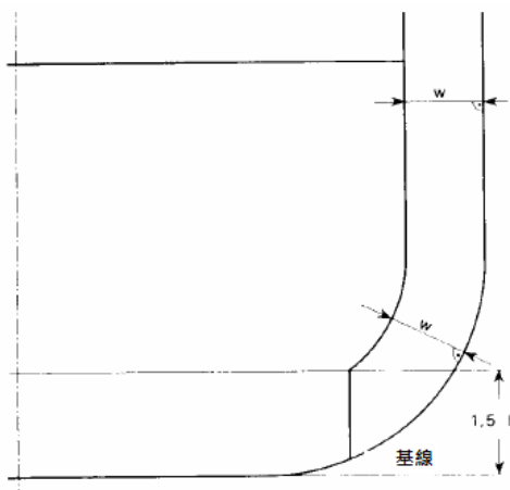
圖 2 - 就本條 2.3.1.4 而言的貨油艙邊界線
