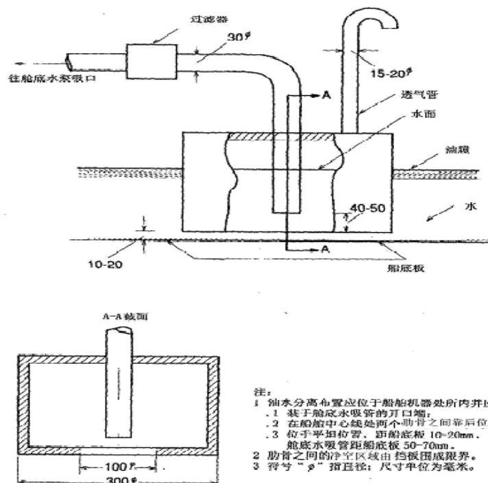
圖 2.2.5.3 (2) - 油水分離佈置 - 僅用於 400 總噸以下的小船
