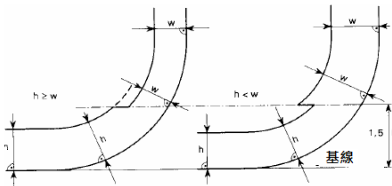
圖 2—關於 2.2.2.7 和 2.2.2.8 的燃油艙邊界線
