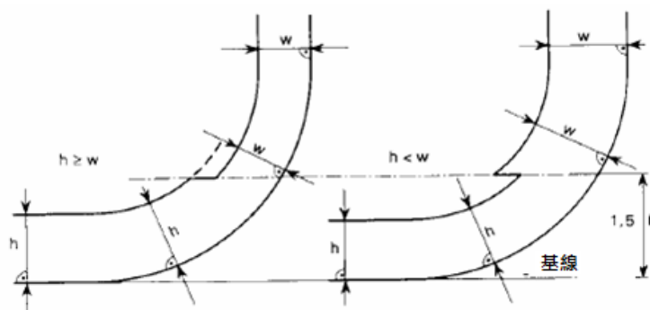
圖 1 - 就本條 2.3.1.3 而言的貨油艙邊界線
