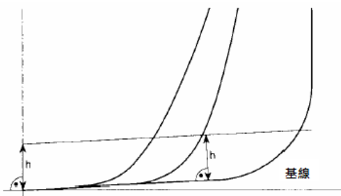
圖 3 – 就本條 2.3.1.6 而言的貨油艙邊界線
