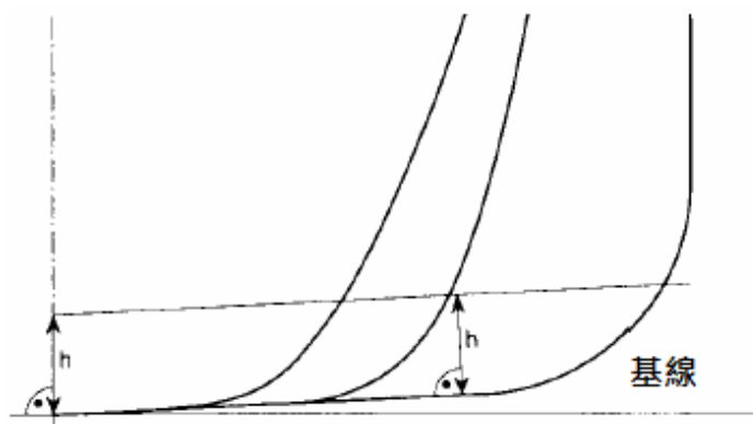
圖 1—關於 2.2.2.6 的燃油艙邊界線
